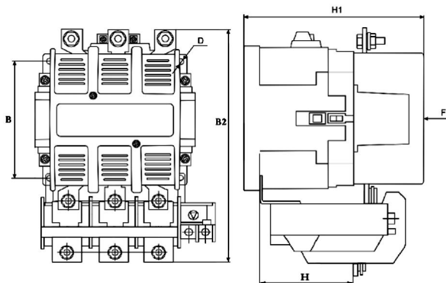
Рисунок 2. Пускатель неревсивного типа с тепловым реле
