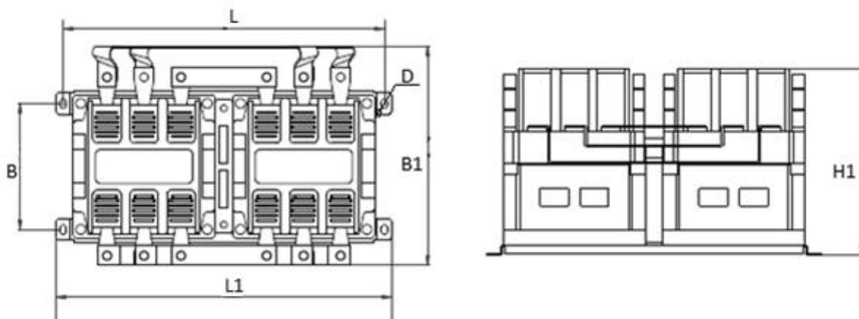
Рисунок 3. Пускатель реверсивного типа
