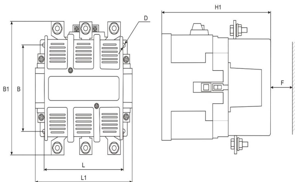
Рисунок 1. Пускатель неревсивного типа
