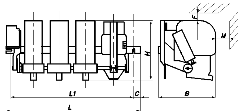
Общий вид и габаритные размеры контакторов серии КТ-6000
