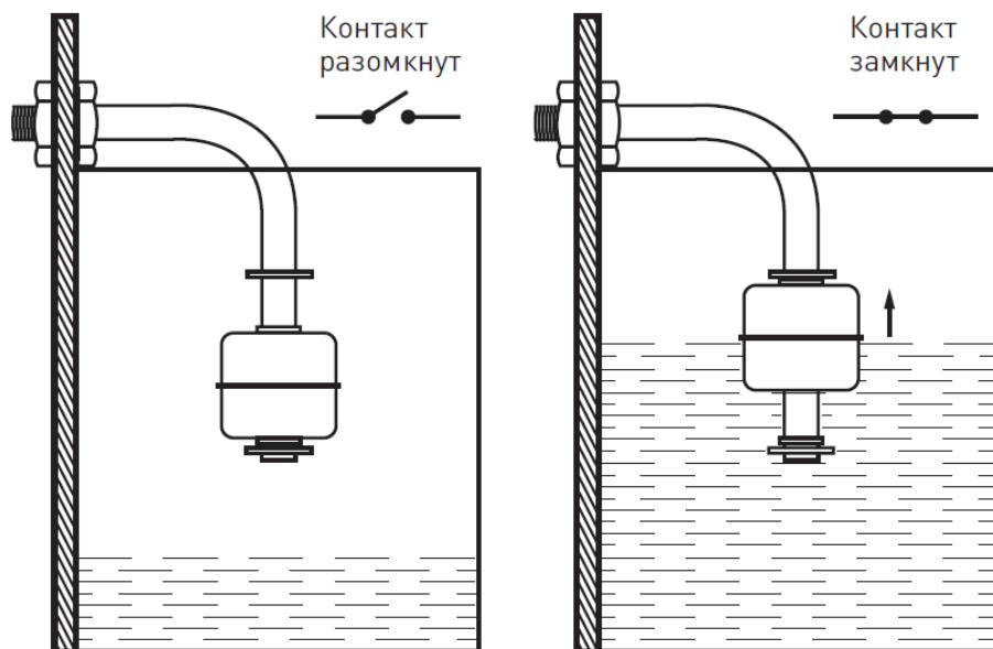
Принцип работы датчика
