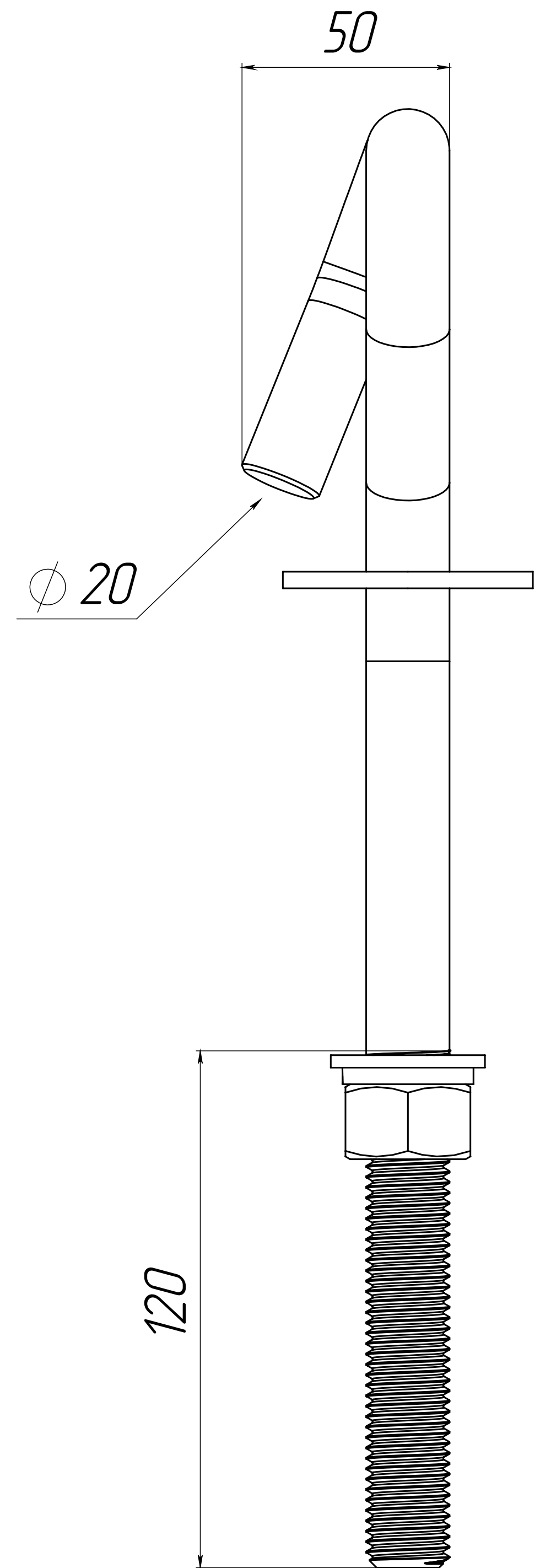
б-20.ГМ Крюк монтажный В20 ЕКФ
