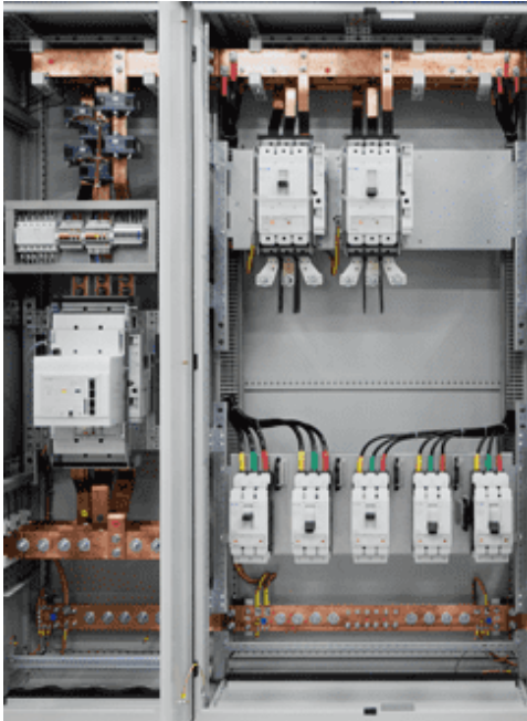
Сборщики НКУ
