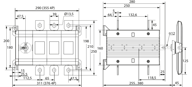
Реверсивный рубильник 630-800 A
