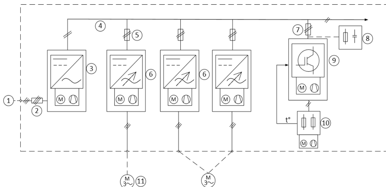
Упрощенная схема подключения тормозного прерывателя в системе привода:
