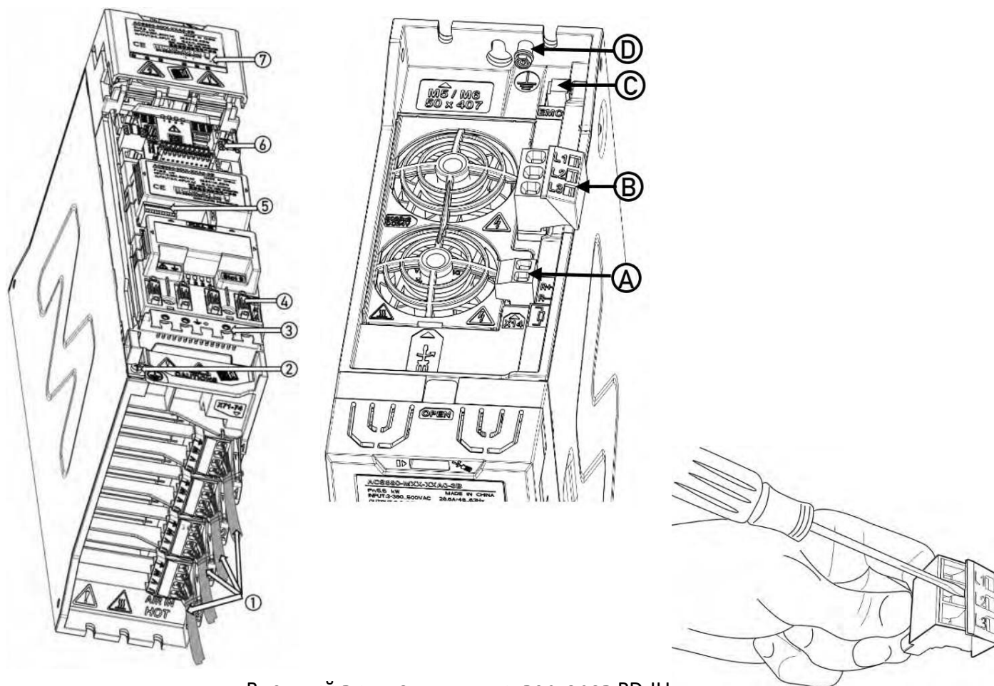
Внешний вид модульных инверторов PD-IU
