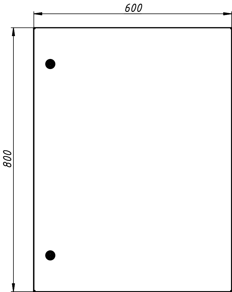
Вид сверху
