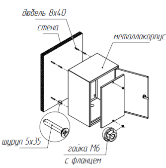
Рис. 1.1. Схема настенного монтажа
