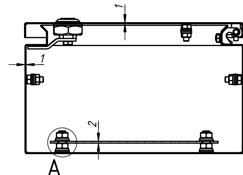
Вид слева
