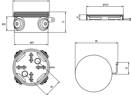
Коробка установочная KMP-050-041
