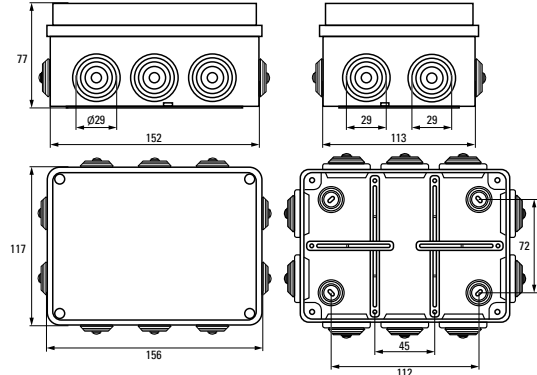
Коробка установочная KMP-050-041
