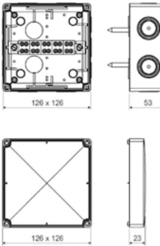
Коробка установочная KMRF-126-506-2
