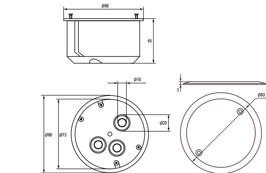
Коробка установочная КМП-020-026
