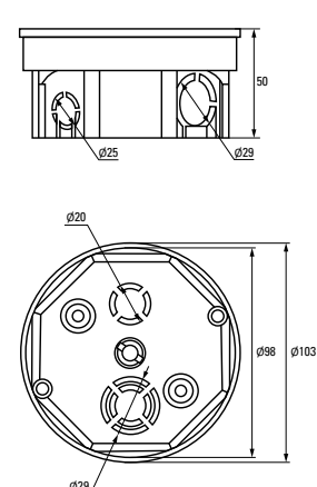
Коробка установочная KMT-010-005
