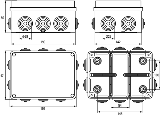
Коробка установочная KMP-050-042
