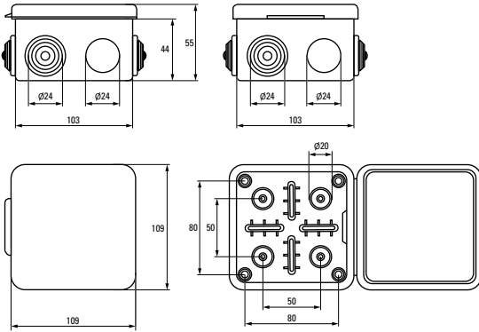
Коробка установочная KMP-030-014
