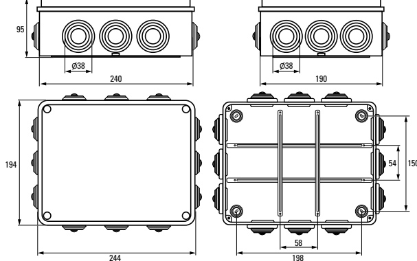
Коробка установочная KMP-050-043
