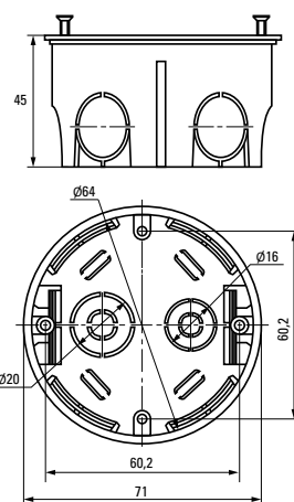
Коробка установочная KMT-010-033
