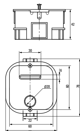
Коробка установочная KMT-010-003
