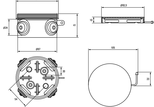
Коробка установочная KMP-050-042
