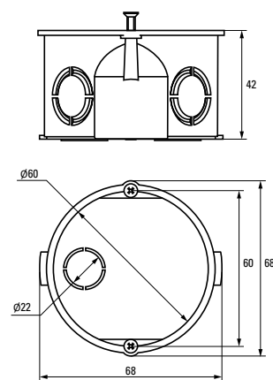
Коробка установочная КМТ-010-001
