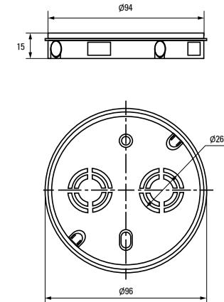
Коробка установочная КМТ-191
