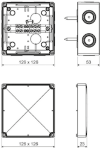
Коробка установочная KMRF-126-506
