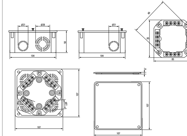
Коробка установочная КМТ-010-022
