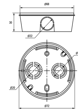
Коробка установочная КМТ-195
