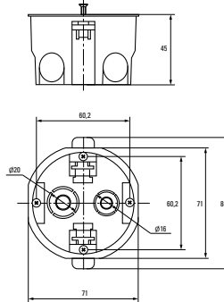
Коробка установочная КМП-020-026
