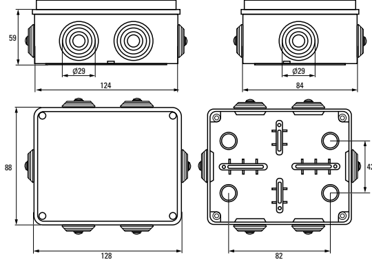
Коробка установочная KMP-050-048
