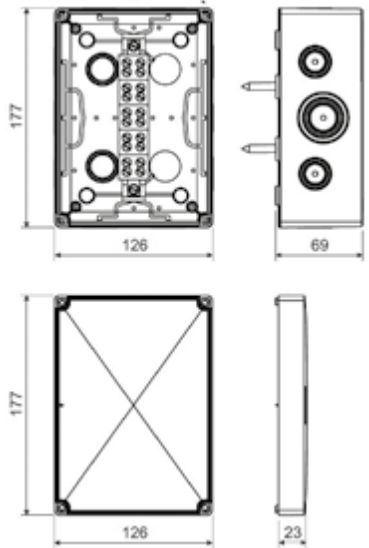
Коробка установочная KMRF-176-516
