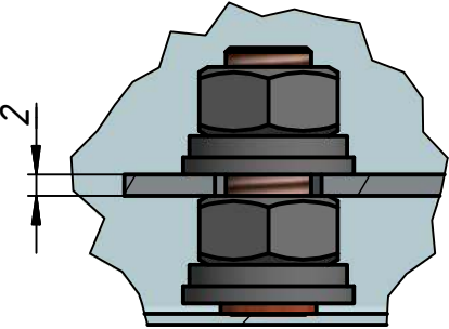
Вид слева
