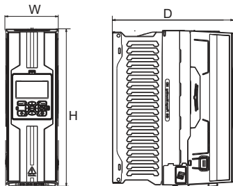
Рис. 1 Габаритные размеры преобразователей частоты PRO-Drive-500 от 1.5 до 11кВт
