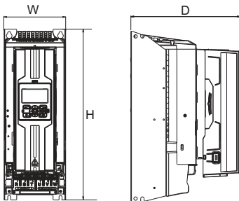
Рис. 2 Габаритные размеры преобразователей частоты PRO-Drive-500 от 15 до 45кВт
