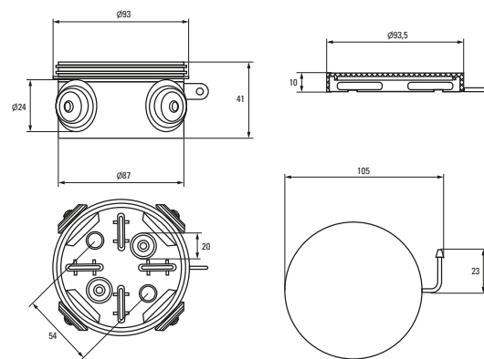
Коробка установочная КМР-050-042
