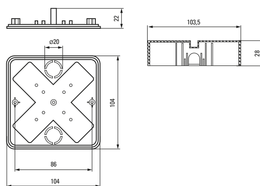
Коробка установочная КМР-030-032 и КМР-030-032kg
