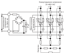
Рис. 7. Схема подключения реле
