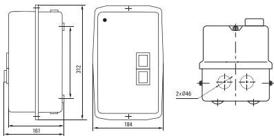
Рис. 3. Габаритные размеры для ПМЛ-3 (40-95А)
