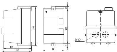
Рис. 2. Габаритные размеры для ПМЛ-2 (25-32А)
