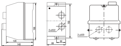
Рис. 1. Габаритные размеры для ПМЛ-1 (9-18А)
