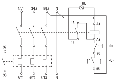
Рис. 7. Схема подключения ПМЛ-3 (40-95А) 400 В
