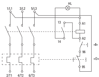
Рис. 4. Схема подключения ПМЛ-1,2 (9-32А) 230 В
