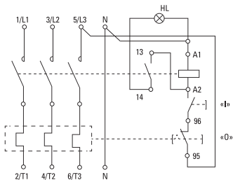
Рис. 6. Схема подключения ПМЛ-3 (40-95А) 230 В
