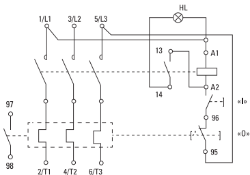
Рис. 5. Схема подключения ПМЛ-1,2 (9-32А) 400 В
