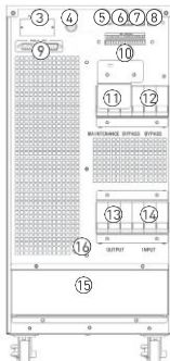
Вид сзади 30кВА
