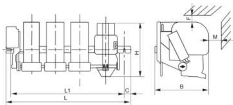
Рис. 1. Габаритные и установочные размеры контакторов КТ-6000 ЕКФ
