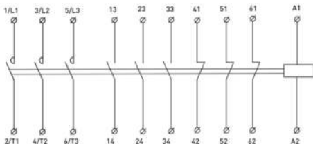
Рис. 2. Схема подключения контактора КТ-6000 ЕКФ
