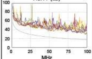
ACR-N (dB)
