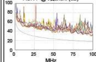
ACR-N @ Удален. (dB)
