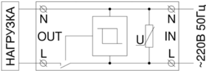
Рисунок 2 – Схема подключения.
