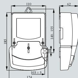
Тип корпуса S34
