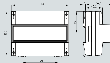
Тип корпуса R32 (P32)
