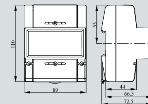
Тип корпуса C36
