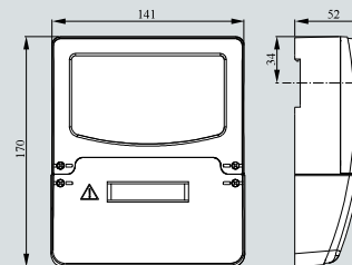
Тип корпуса R32 (P32)
