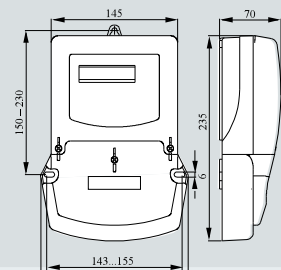
Тип корпуса S33 (Ш33)
