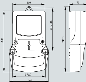
Тип корпуса S10
