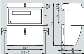
Тип корпуса S32
