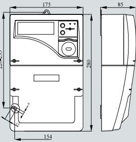
Тип корпуса S34
