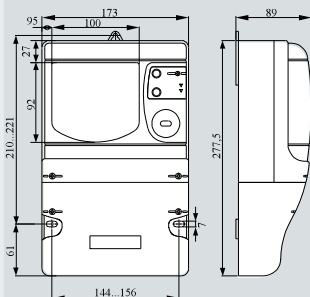
Тип корпуса S32
