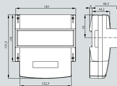
Тип корпуса R33
