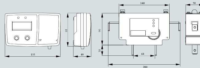
Тип корпуса C2
