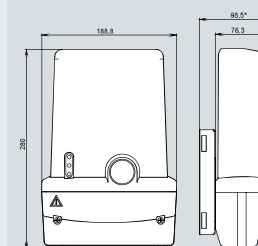
Тип корпуса C36
