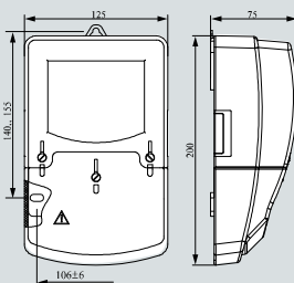
Тип корпуса S8
