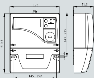
Тип корпуса S31 (Ш31)
