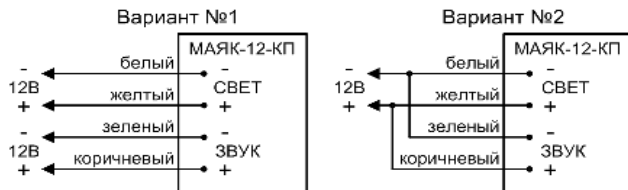
Рис.1 Схема подключения.
