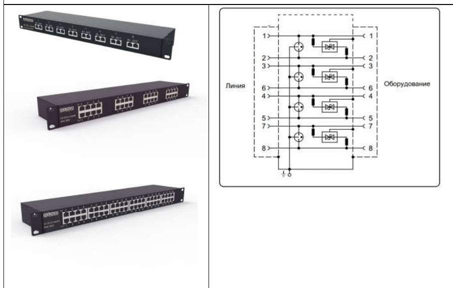
Рис.5 Внешний вид и электрическая схема SP-IP8/1000(ver.2)
