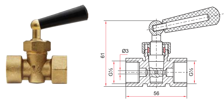
Трехходовой кран Watts
