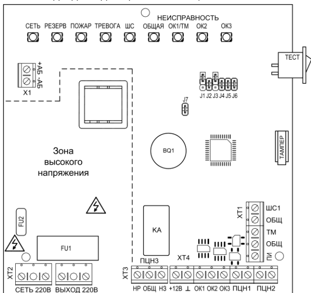
Рис.3 Плата прибора
