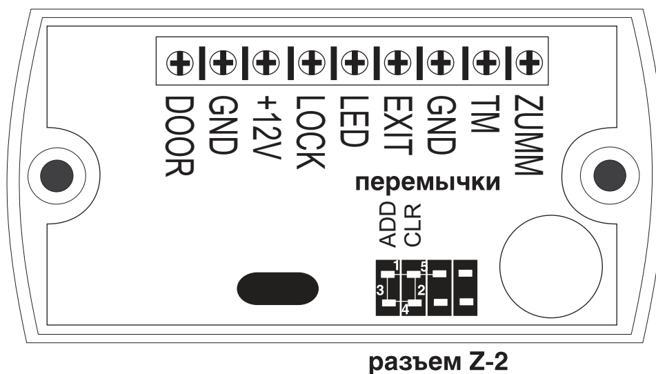
Рис. 3 Положение перемычек
