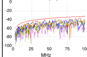
ACR-F (dB)
