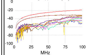
ACR-N @ Удален. (dB)
