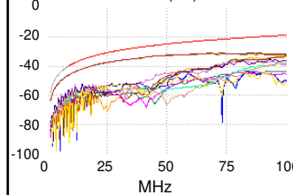
ACR-N (dB)
