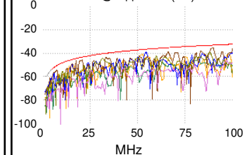
ACR-F @ Удален. (dB)
