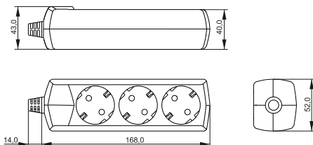
Рисунок 1 – Колодка удлинителя У03
