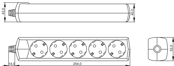
Рисунок 2 – Колодка удлинителя У05
