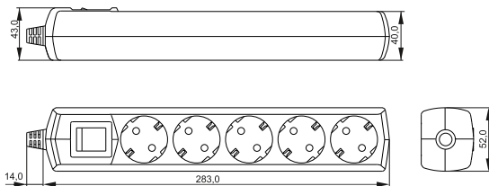
Рисунок 4 – Колodka удлинителя У05В
