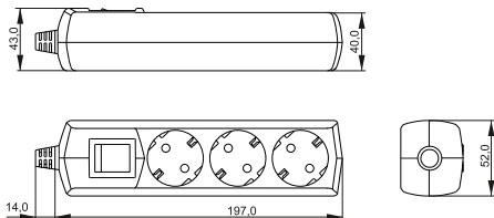
Рисунок 3 – Колodka удлинителя У03В
