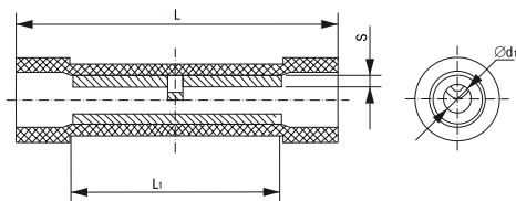
Рисунок 1 – Гильза ГСИ, ГСИ-н
