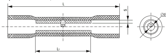
Рисунок 2 – Гильза ГСИ-т
