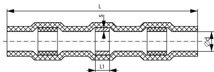
Рисунок 3 – Гильза ГСИ-п
