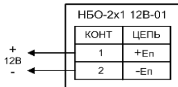
Рис.1 Схема подключения.
