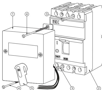
Рис. 3 Схема монтажа электроприводов ЭП-32/33
