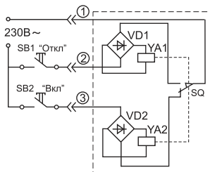
Рис. 2 Схема электрическая принципиальная
