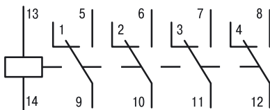
Рисунок 2. Электрические схемы реле РЭК77, РЭК78
