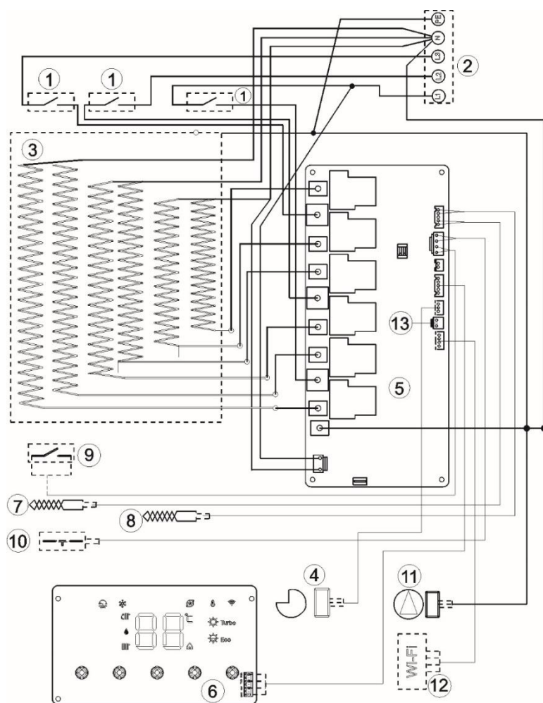
Рис. 16. Электрическая схема THERMEX Boss 12 Wi-Fi
