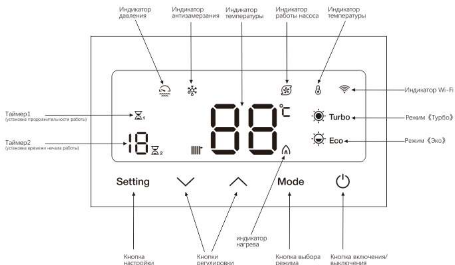
Рис. 3. Панель управления
