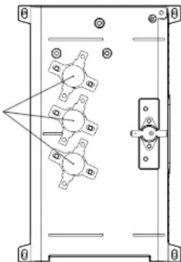
Рис. 19. Ручное восстановление термостатов
