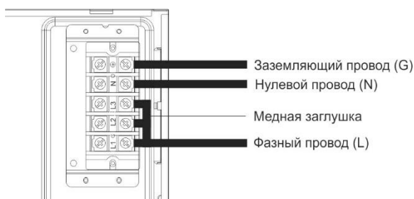
Рис 13. Однофазное подключение прибора
