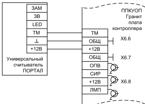
Рис.Б4 Схема подключения универсального считывателя «Портал»
