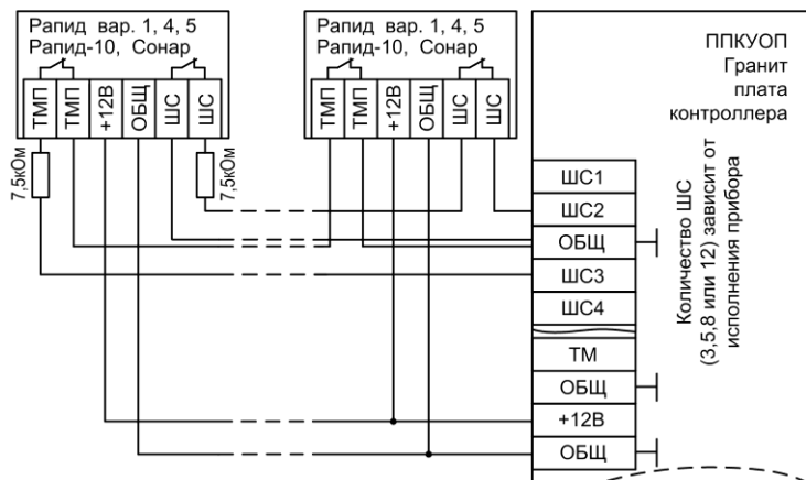
Рис.Б3 Схема подключения охранных извещателей Репид вар.1,4,5, Репид-10, Сонар (тампер подключён к отдельному ШС)
