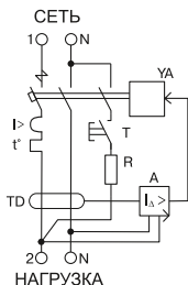
Рисунок 2 – Схема электрическая принципиальная
