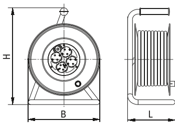
Рисунок 1 – Удлинитель
