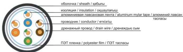
Рисунок 4 – Конструкция кабеля типа F/UTP
