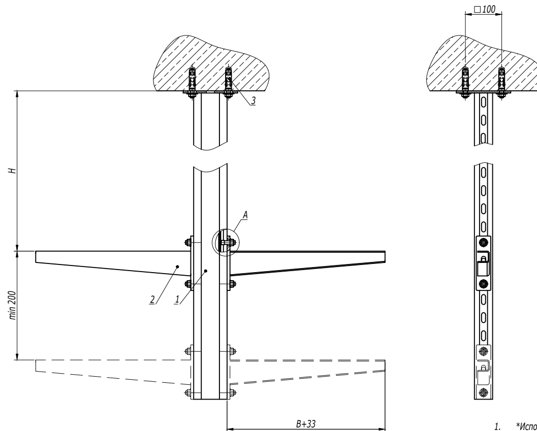
Подвес BSD-92
