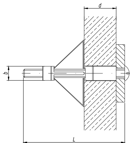
Металлический дюбель для пустотелых конструкций (тип 7)
