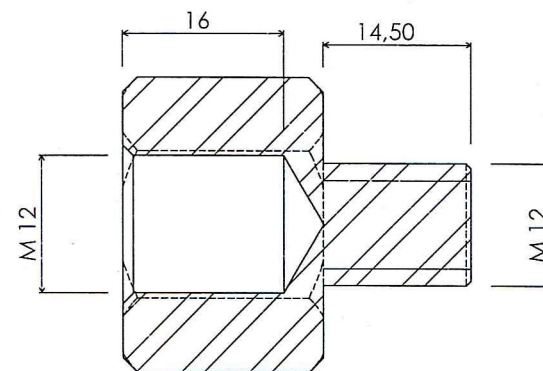
A-A Масштаб 2:1
