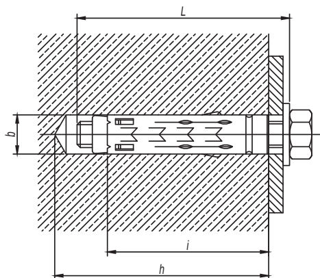
Анкер стандартный с болтом (тип 1)
