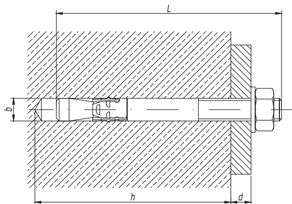
Усиленный клиновой анкер (тип 7)
