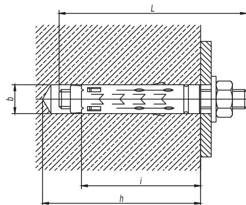
Анкер стандартный со шпилькой (тип 2)
