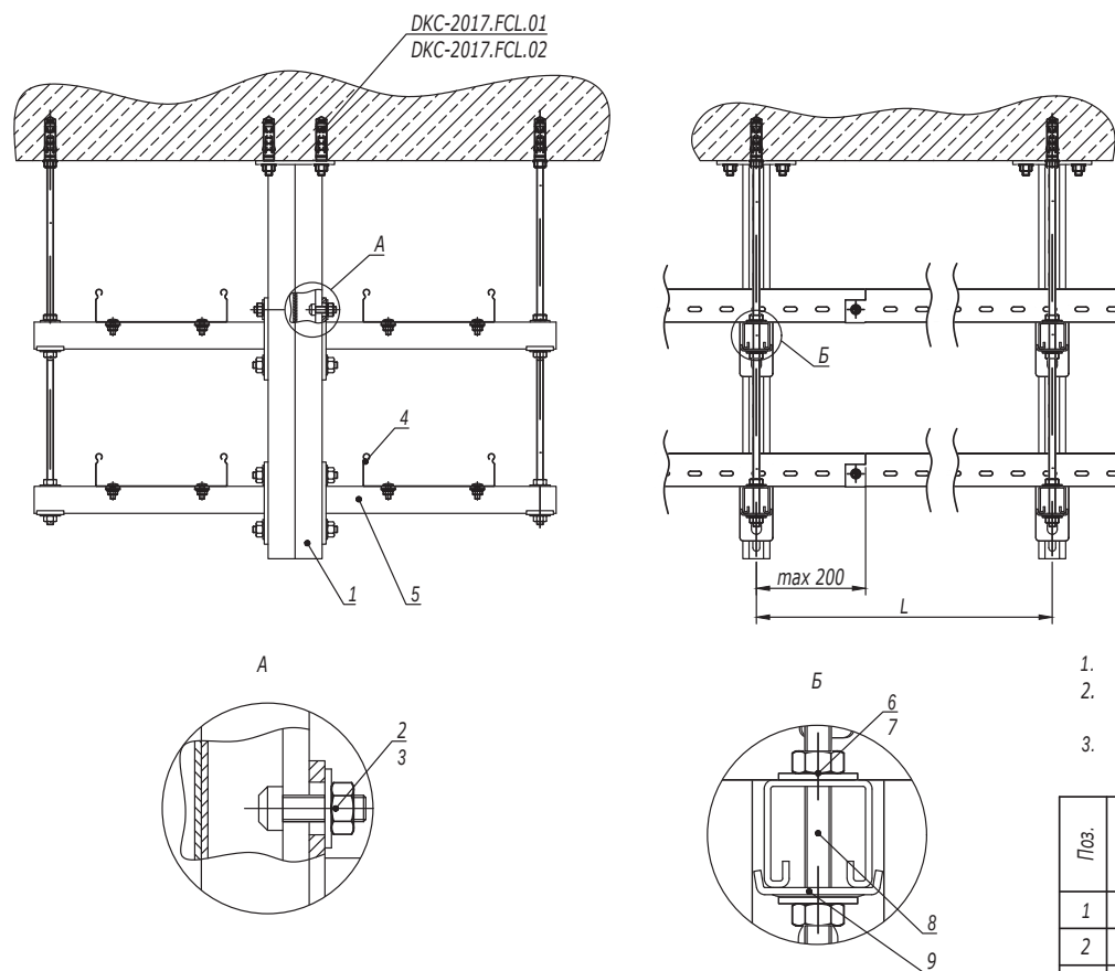
Двусторонняя схема подвеса
