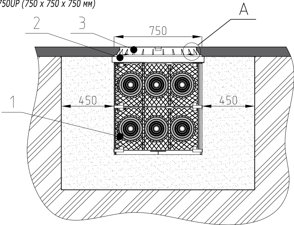
Кабельный колодец 270750UP (750 x 750 x 750 мм)
