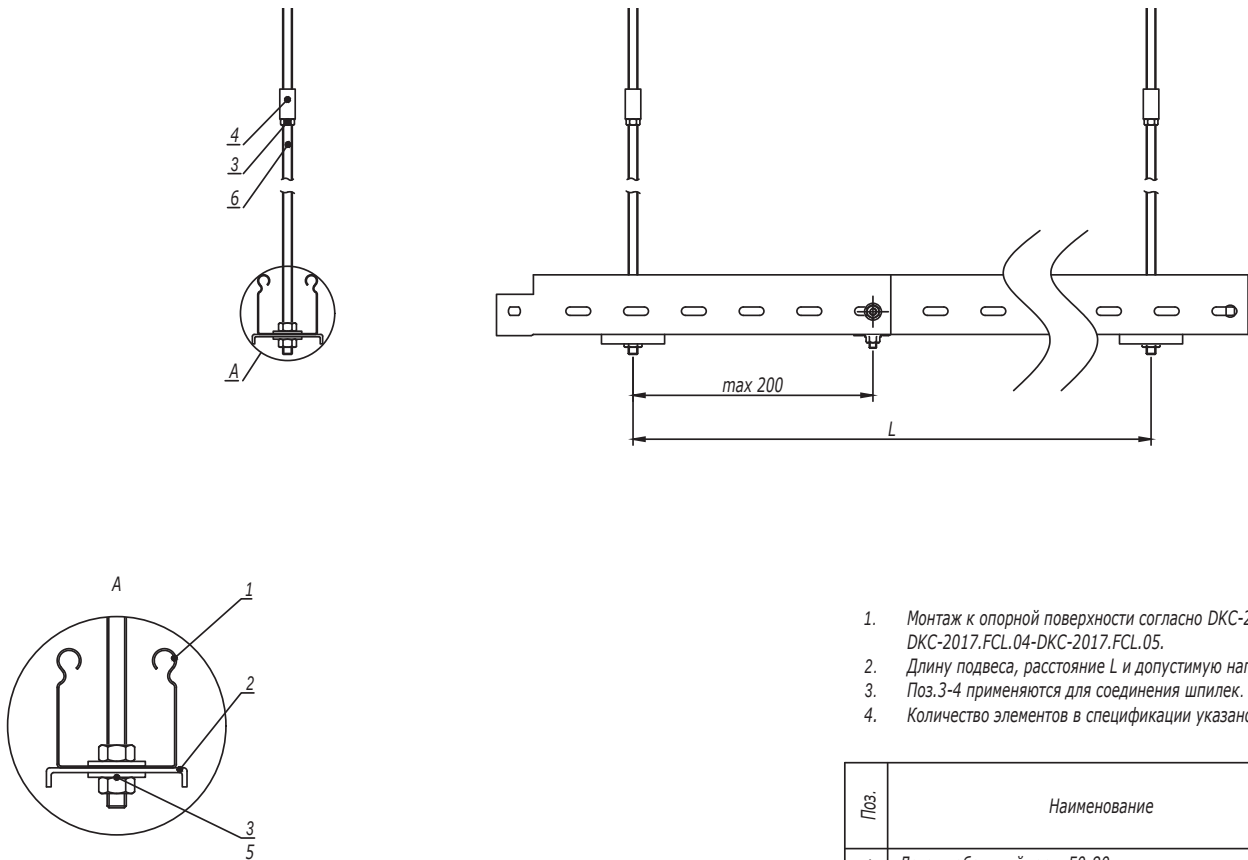
Крепление листового лотка шириной 50-80 мм
