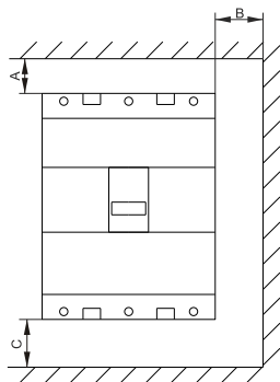
а) минимальные расстояния установки выключателей в щите / the minimum installation distances of the circuit breakers in the switchboard
