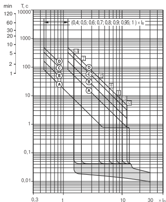
Рисунок 2 – Временнoвые характеристики выключателей с электронным расцепителем / Figure 2 – Time-current characteristics of circuit breakers with electronic release MP211
