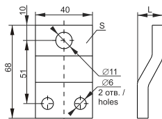
а) наконечник-переходник для / adapter lugs for BA88-35
