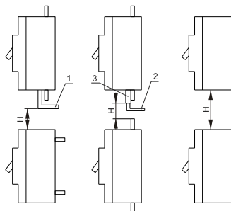
1 – не изолированное присоединение / non insulated connection; 2 – изолированный кабель / insulated cable; 3 – кабельные наконечники / cable lugs
