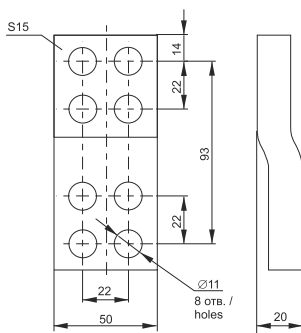
г) наконечник-переходник для / adapter lugs for BA88-43
