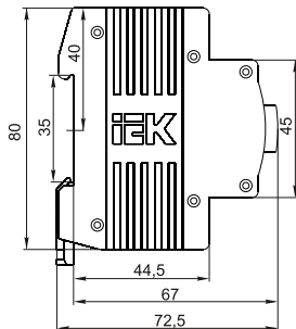
Рисунок 1 – Габаритные размеры / Figure 1 – Overall dimensions
