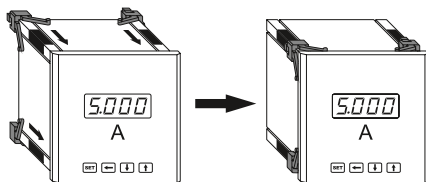
Рисунок 3 – Схема крепления фиксаторов на корпус / Figure 3 - Scheme of fixing the clips on the case
