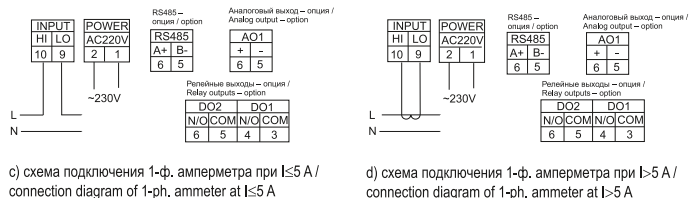
Рисунок 2 – Схемы подключения амперметров и вольтметров / Figure 2 - Connection diagrams of ammeters and voltmeters
