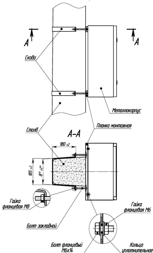
Рисунок 1 — Крепление скобами
